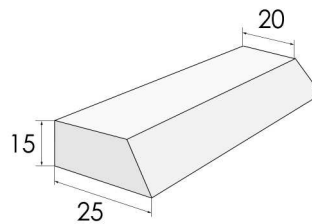
Mineralit Trapezaufkantung
